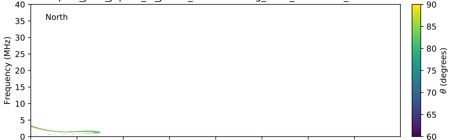
expres_juno_jupiter_io_jrm09_lossc-wid1deg_3kev_20210320_v11.cdf
