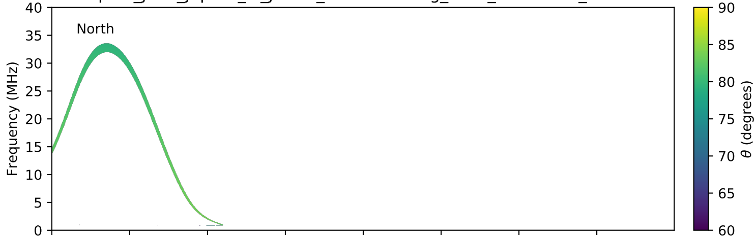
expres_juno_jupiter_io_jrm09_lossc-wid1deg_3kev_20210311_v11.cdf
