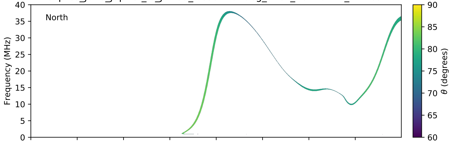
expres_juno_jupiter_io_jrm09_lossc-wid1deg_3kev_20210217_v11.cdf
