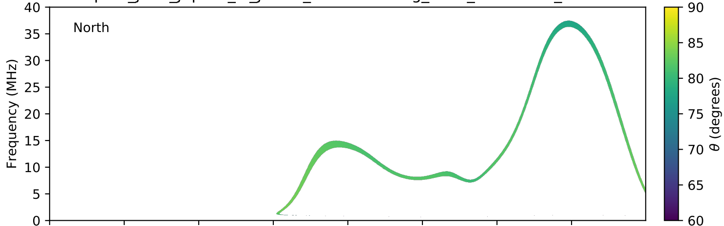
expres_juno_jupiter_io_jrm09_lossc-wid1deg_3kev_20210201_v11.cdf
