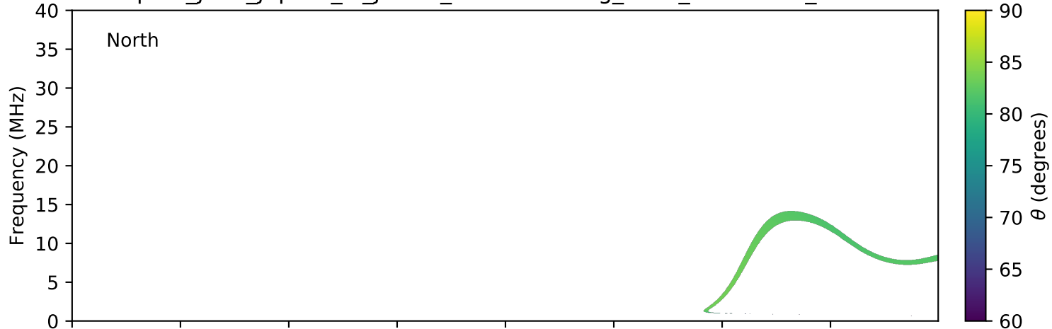
expres_juno_jupiter_io_jrm09_lossc-wid1deg_3kev_20210130_v11.cdf
