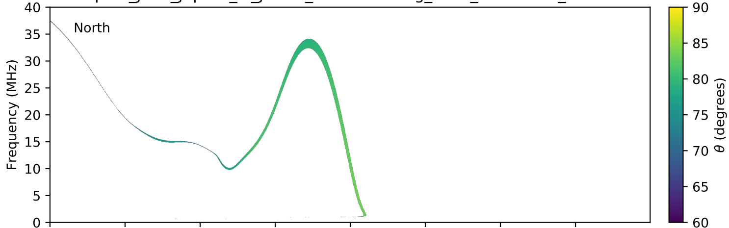
expres_juno_jupiter_io_jrm09_lossc-wid1deg_3kev_20190713_v01.cdf
