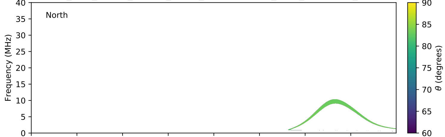
expres_juno_jupiter_europa_jrm09_lossc-wid1deg_3kev_20190725_v01.cdf
