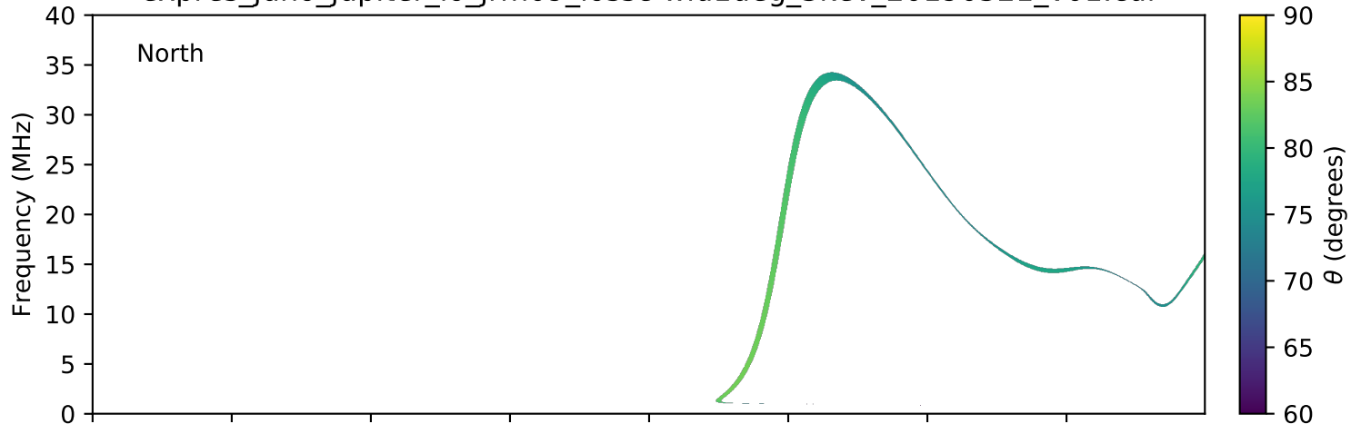
expres_juno_jupiter_io_jrm09_lossc-wid1deg_3kev_20190321_v01.cdf
