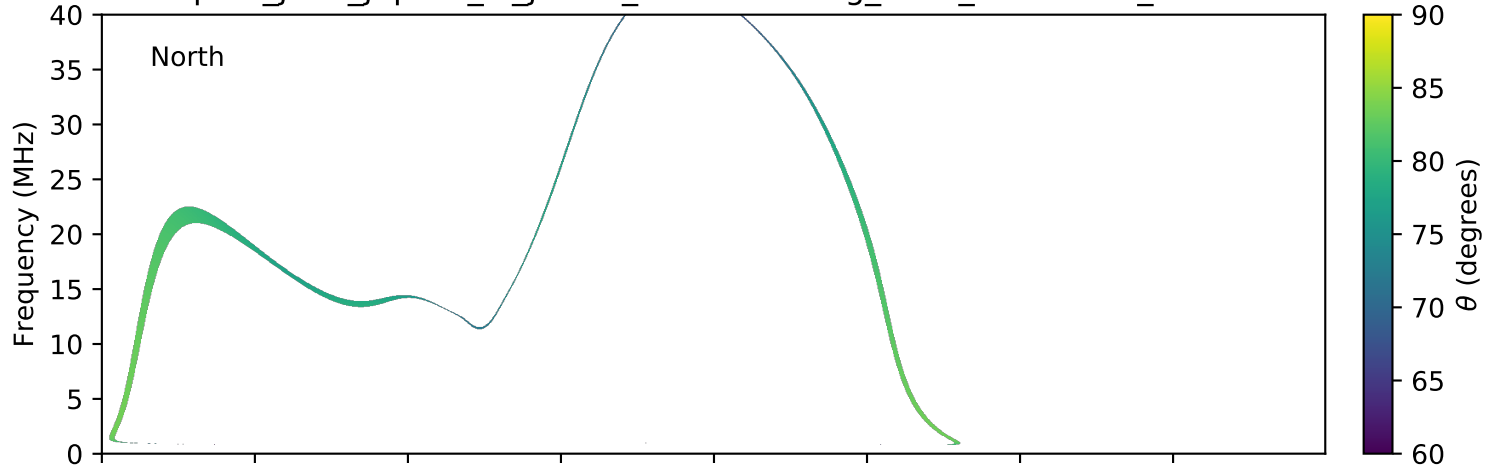
expres_juno_jupiter_io_jrm09_lossc-wid1deg_3kev_20190131_v01.cdf
