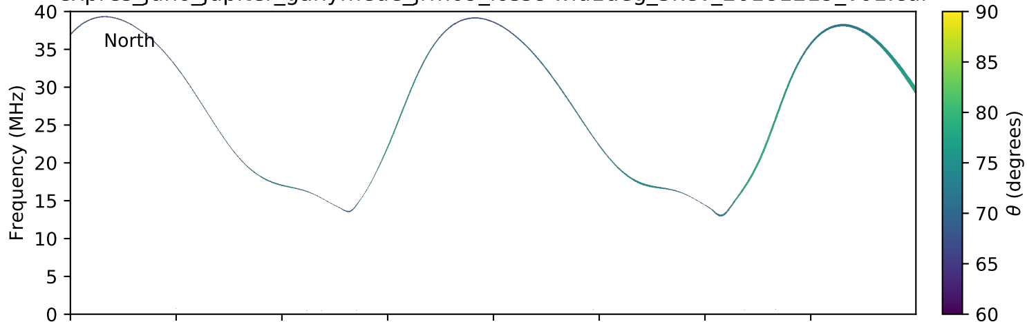
expres_juno_jupiter_ganymede_jrm09_lossc-wid1deg_3kev_20181219_v01.cdf
