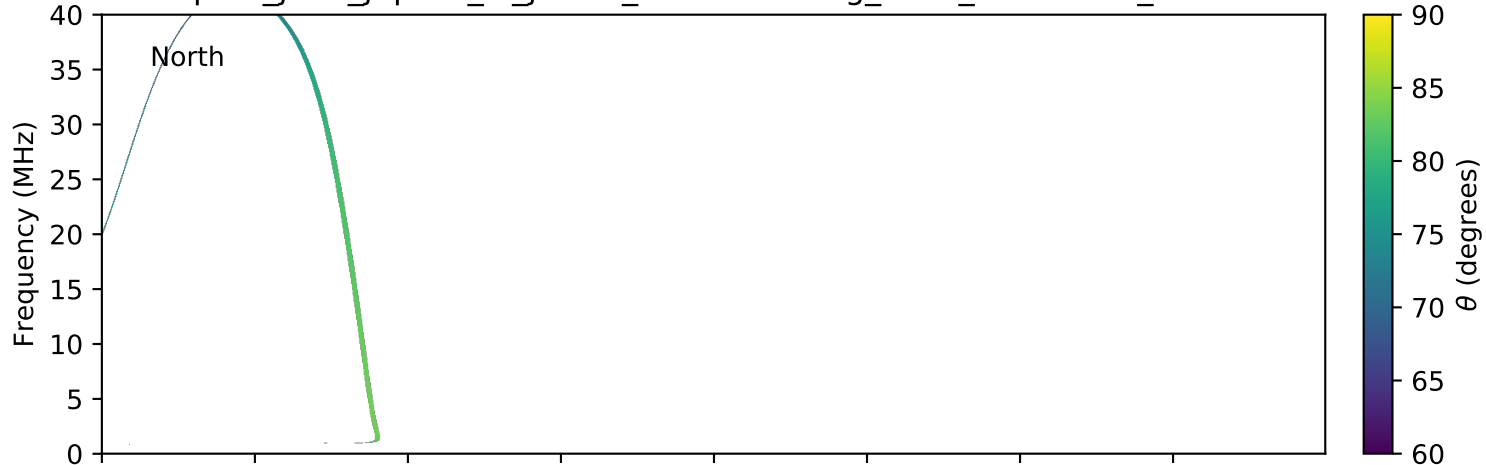
expres_juno_jupiter_io_jrm09_lossc-wid1deg_3kev_20180520_v01.cdf
