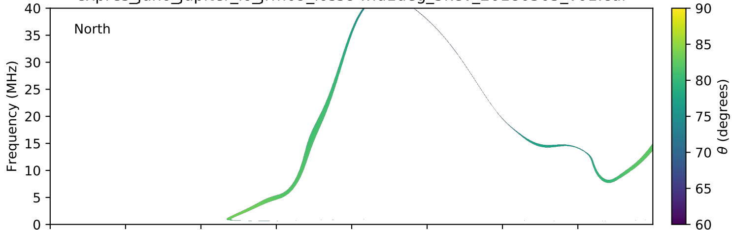
expres_juno_jupiter_io_jrm09_lossc-wid1deg_3kev_20180505_v01.cdf
