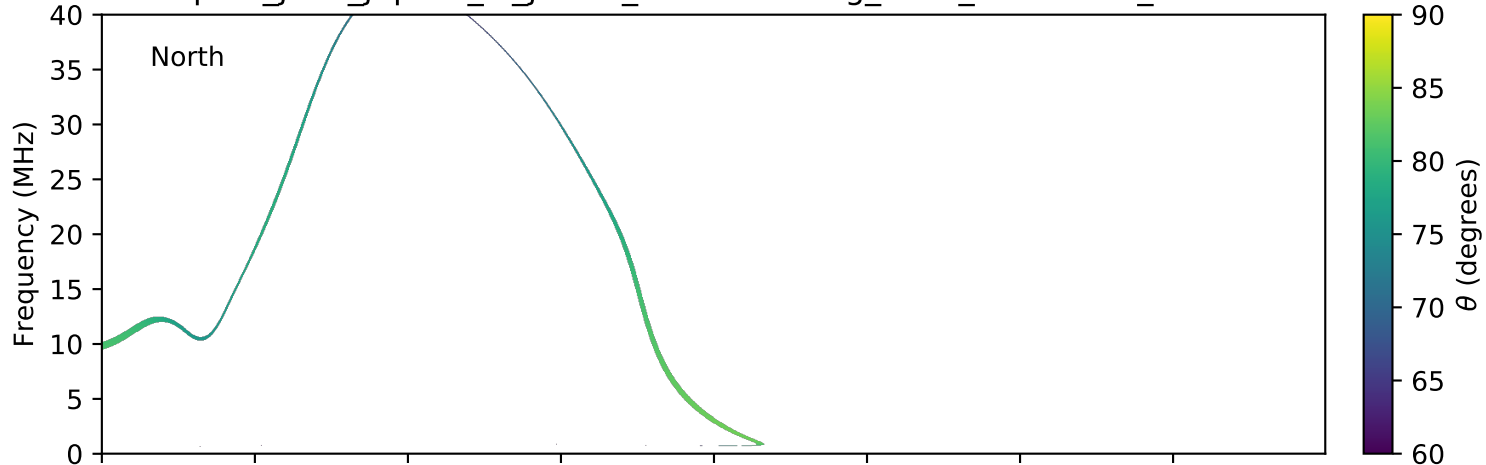
expres_juno_jupiter_io_jrm09_lossc-wid1deg_3kev_20180301_v01.cdf
