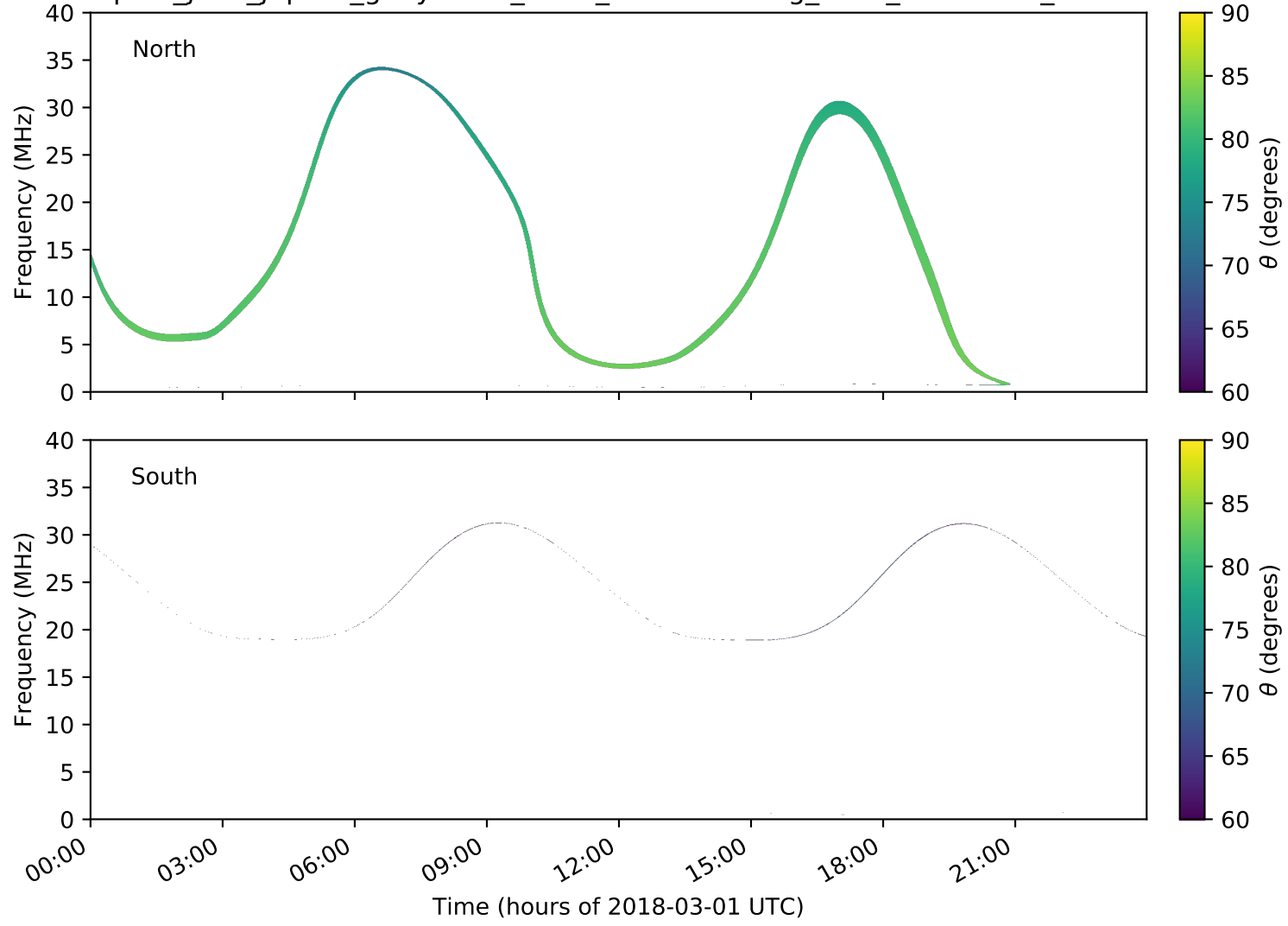
expres_juno_jupiter_ganymede_isaac_lossc-wid1deg_3kev_20180301_v01.cdf
