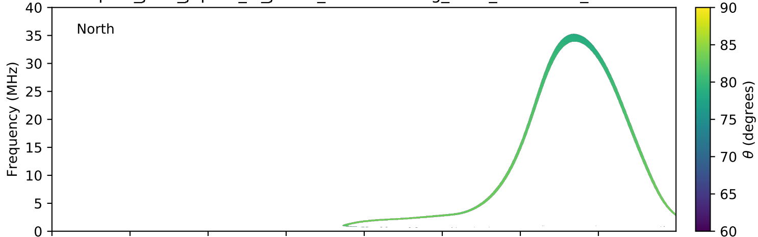
expres_juno_jupiter_io_jrm09_lossc-wid1deg_3kev_20180209_v01.cdf
