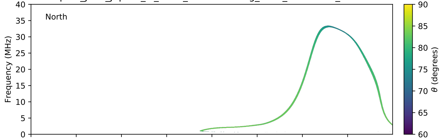
expres_juno_jupiter_io_isaac_lossc-wid1deg_3kev_20180209_v01.cdf
