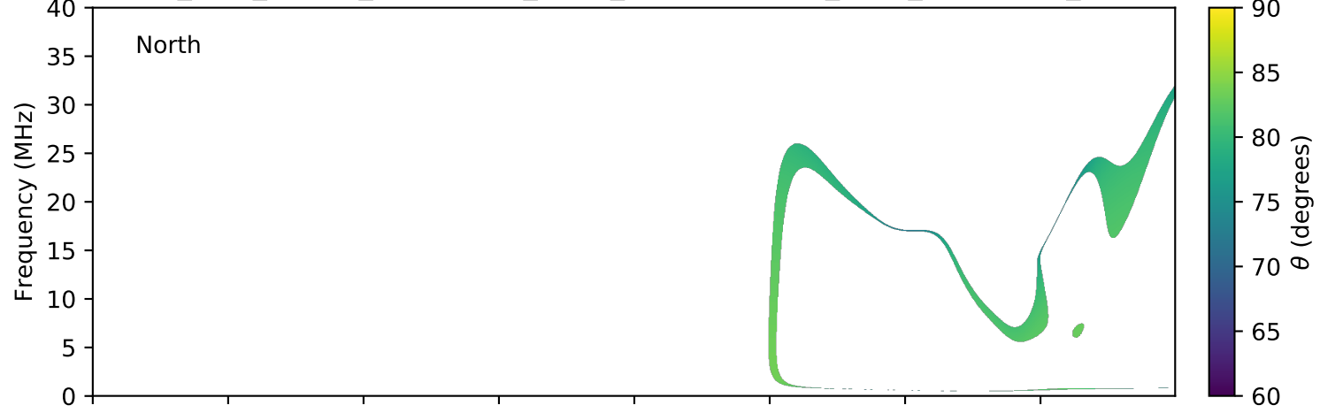
expres_juno_jupiter_ganymede_isaac_lossc-wid1deg_3kev_20180205_v01.cdf
