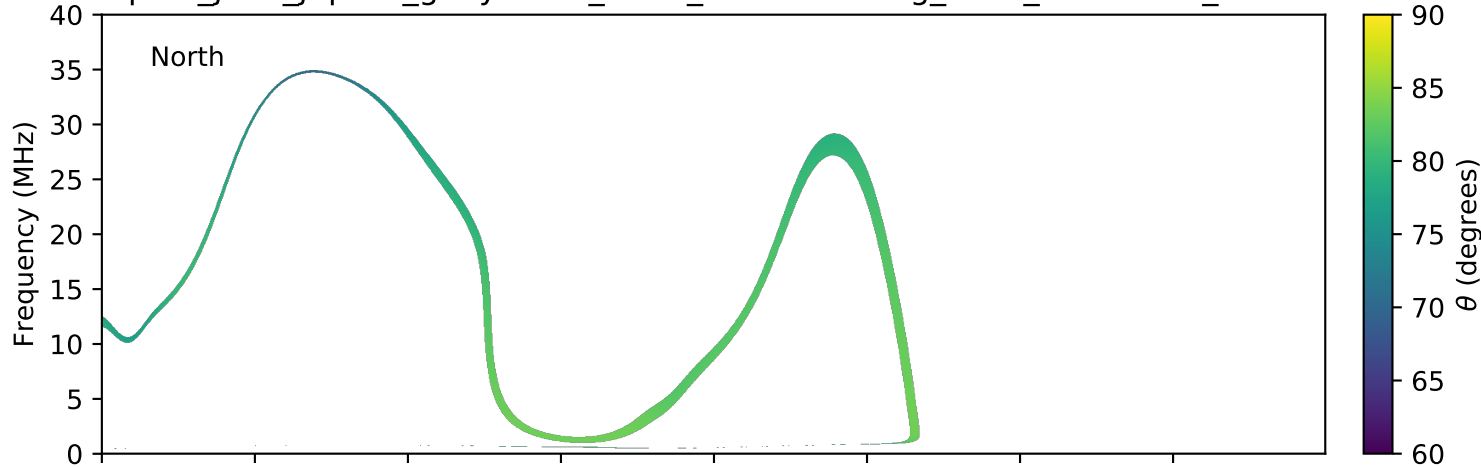
expres_juno_jupiter_ganymede_isaac_lossc-wid1deg_3kev_20180201_v01.cdf
