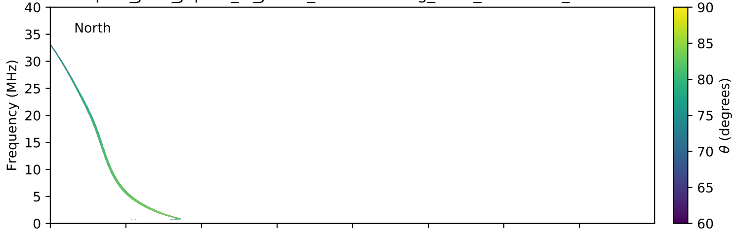
expres_juno_jupiter_io_jrm09_lossc-wid1deg_3kev_20171101_v01.cdf
