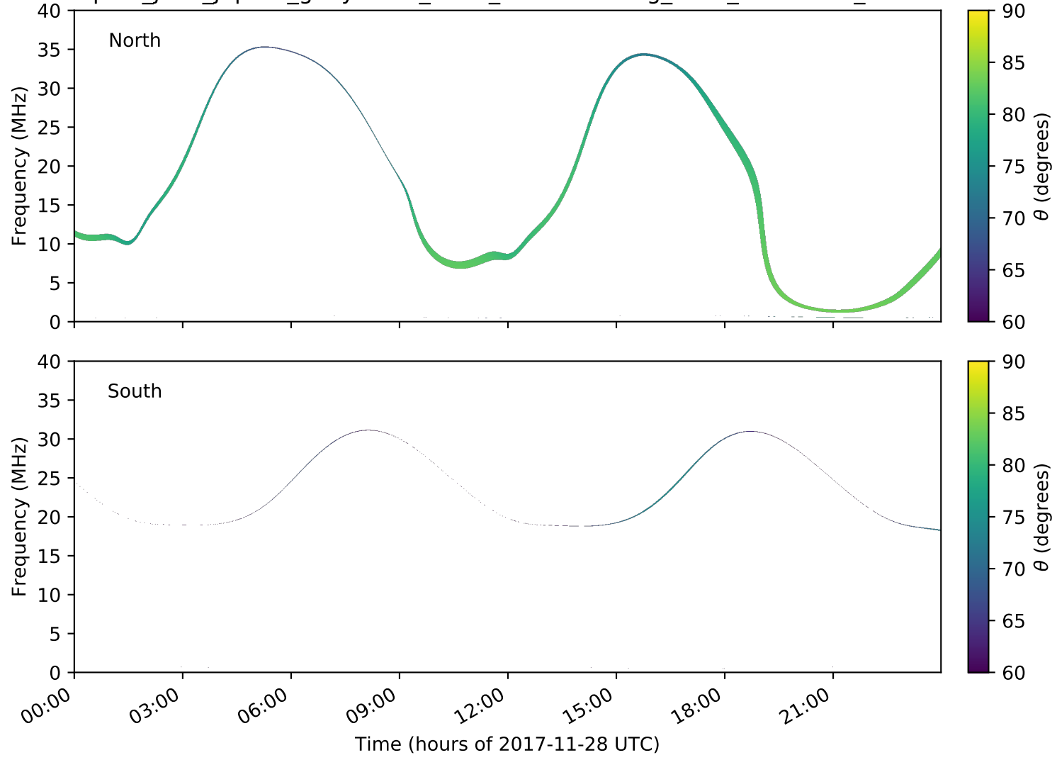
expres_juno_jupiter_ganymede_isaac_lossc-wid1deg_3kev_20171128_v01.cdf
