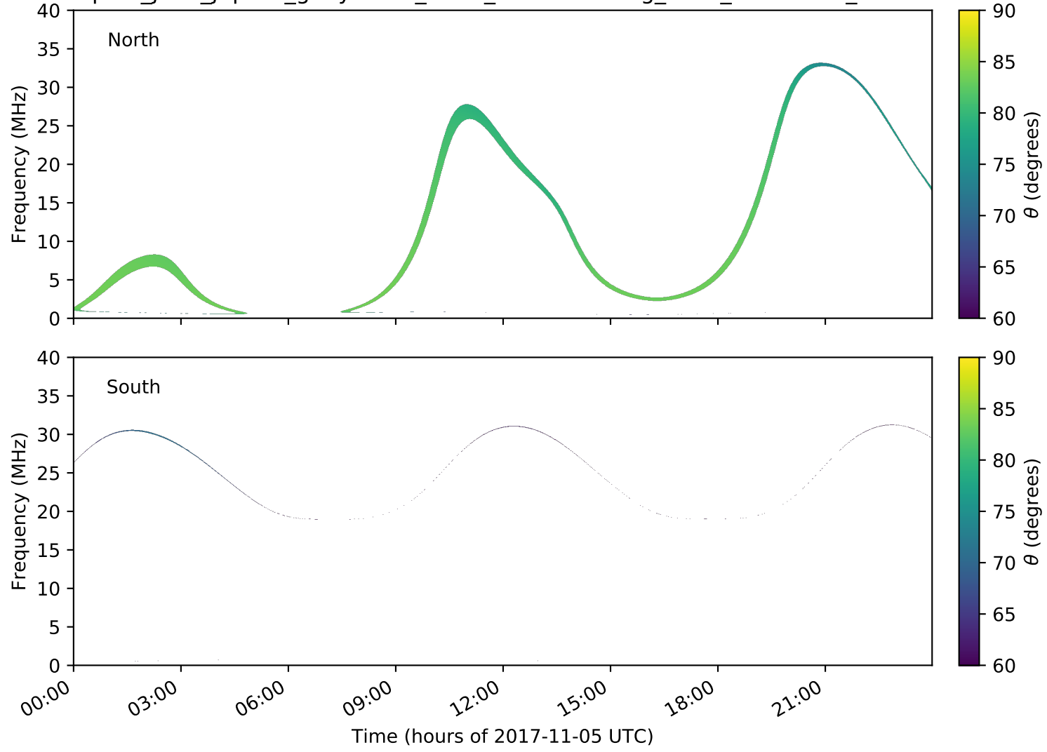
expres_juno_jupiter_ganymede_isaac_lossc-wid1deg_3kev_20171105_v01.cdf
