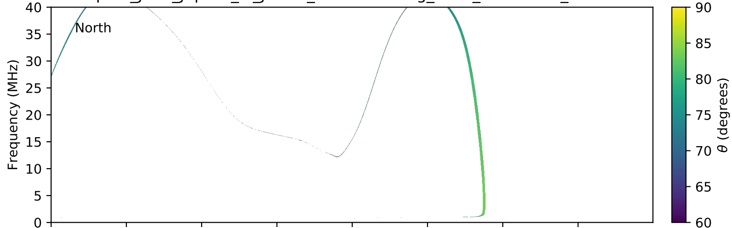
expres_juno_jupiter_io_jrm09_lossc-wid1deg_3kev_20171021_v01.cdf
