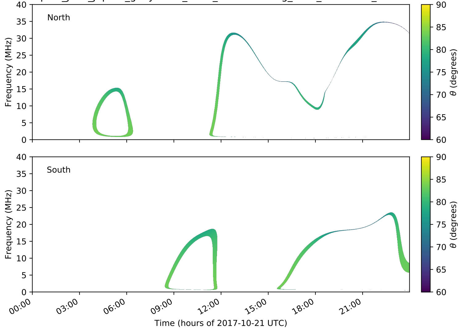
expres_juno_jupiter_ganymede_isaac_lossc-wid1deg_3kev_20171021_v01.cdf
