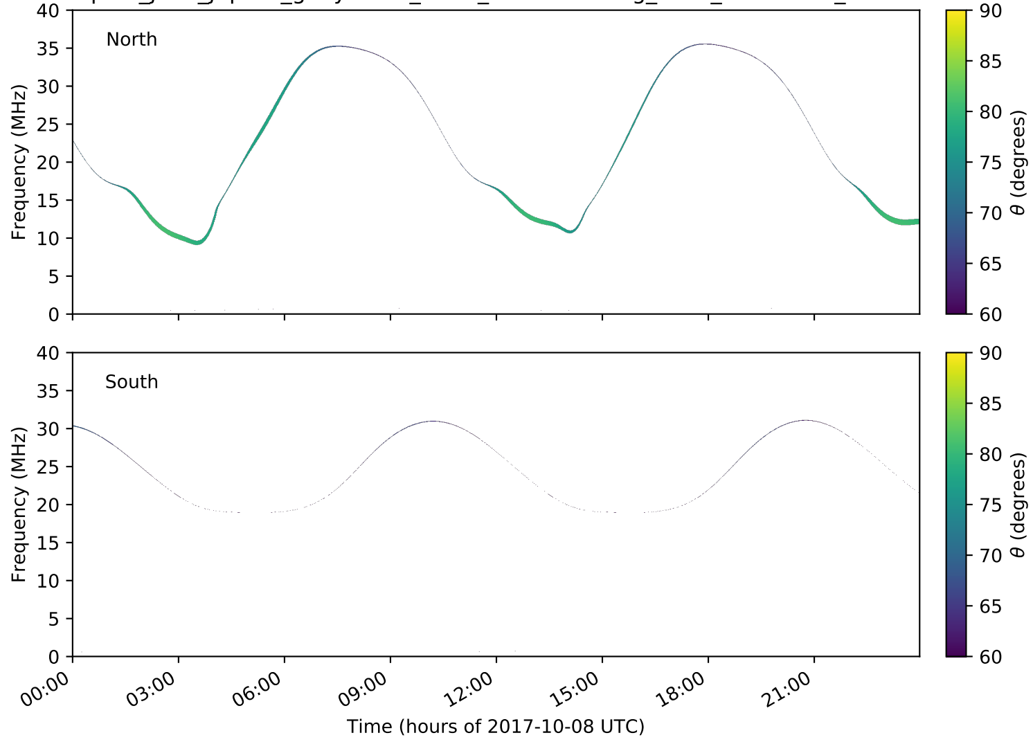
expres_juno_jupiter_ganymede_isaac_lossc-wid1deg_3kev_20171008_v01.cdf
