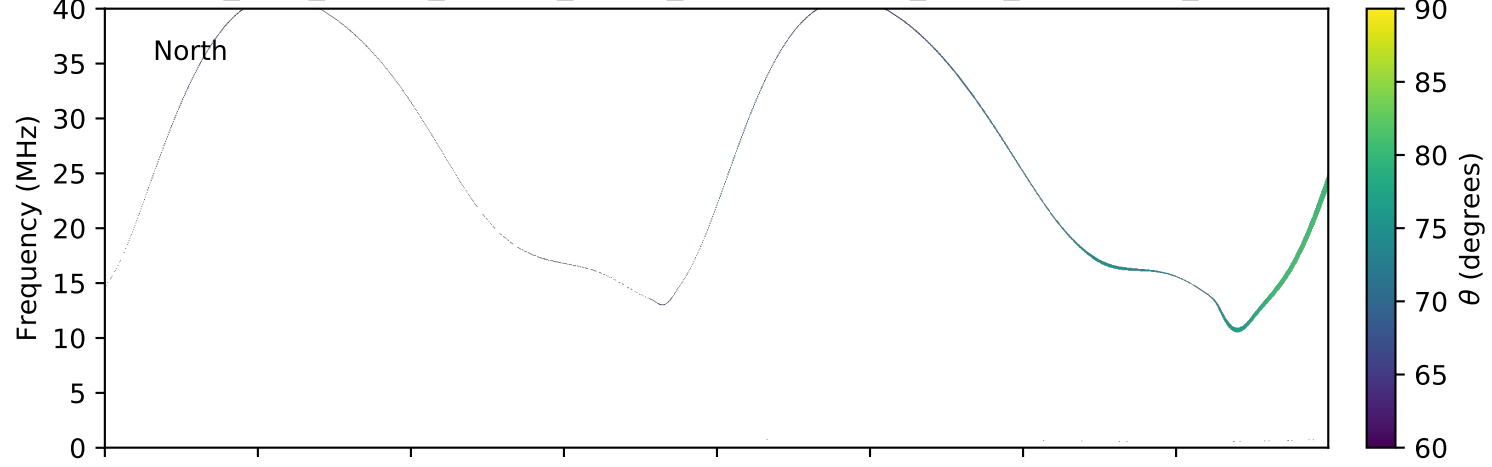
expres_juno_jupiter_europa_jrm09_lossc-wid1deg_3kev_20171021_v01.cdf
