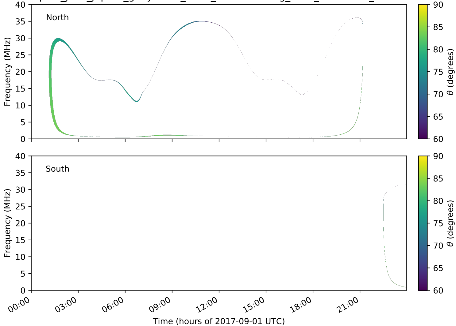
expres_juno_jupiter_ganymede_isaac_lossc-wid1deg_3kev_20170901_v01.cdf
