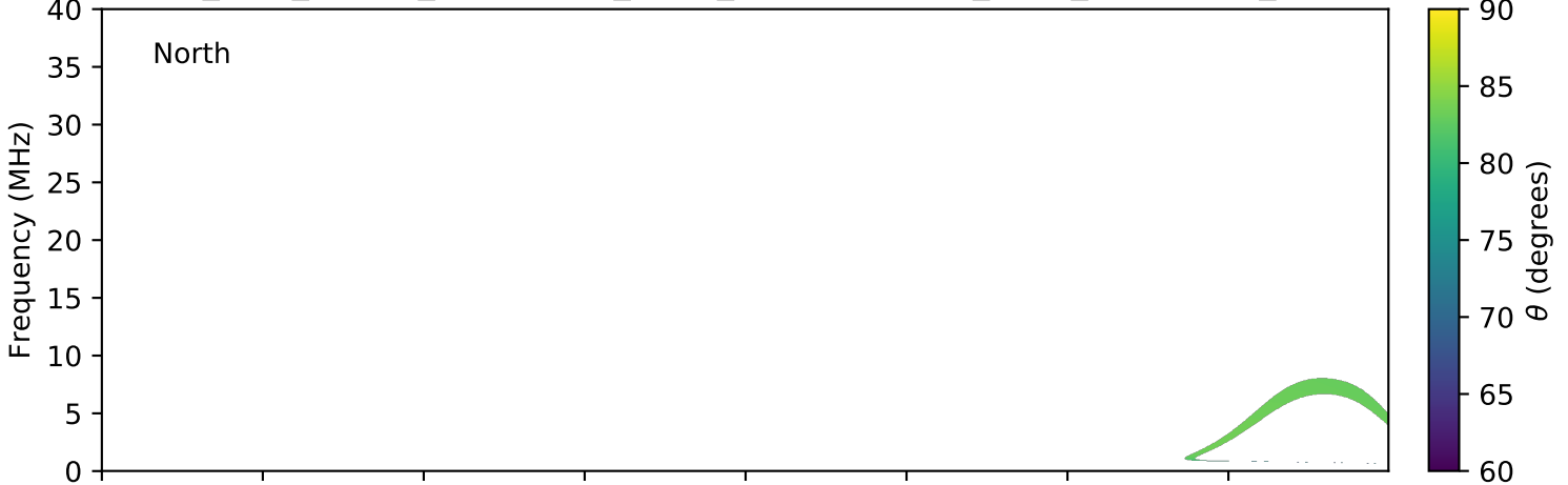
expres_juno_jupiter_ganymede_isaac_lossc-wid1deg_3kev_20170713_v01.cdf
