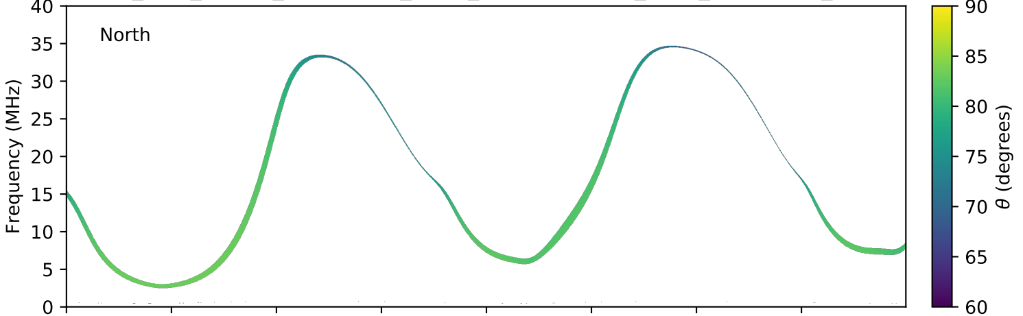
expres_juno_jupiter_ganymede_isaac_lossc-wid1deg_3kev_20170601_v01.cdf
