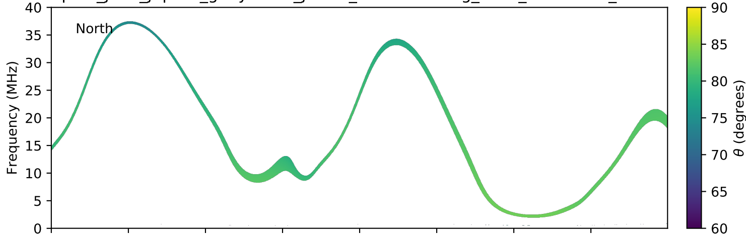
expres_juno_jupiter_ganymede_jrm09_lossc-wid1deg_3kev_20170413_v01.cdf
