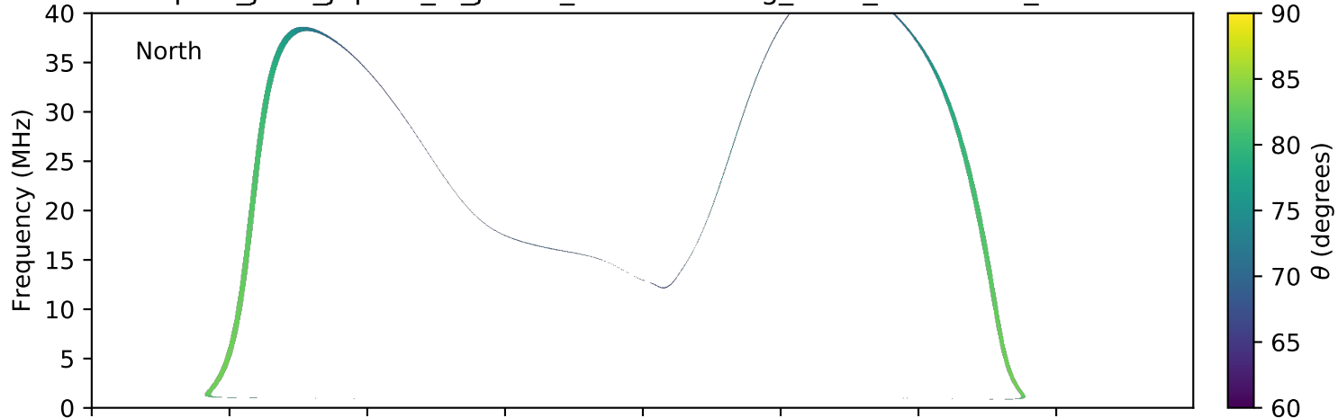
expres_juno_jupiter_io_jrm09_lossc-wid1deg_3kev_20170109_v01.cdf
