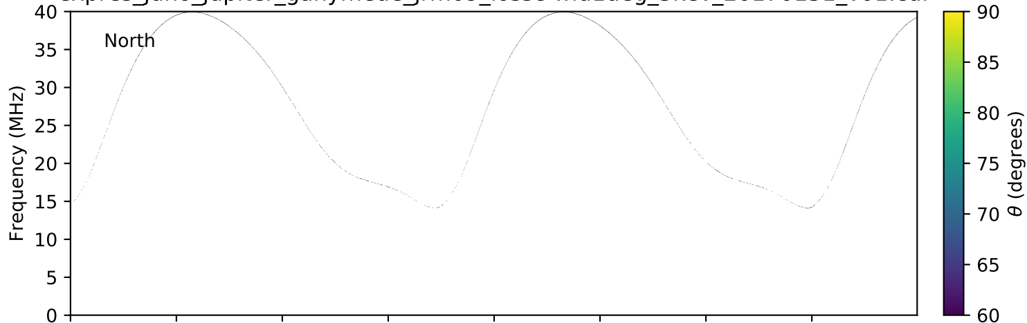
expres_juno_jupiter_ganymede_jrm09_lossc-wid1deg_3kev_20170131_v01.cdf
