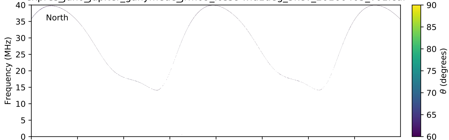
expres_juno_jupiter_ganymede_jrm09_lossc-wid1deg_3kev_20160405_v01.cdf
