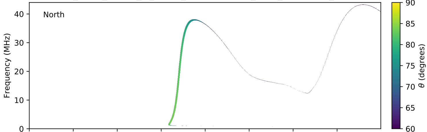
expres_earth_jupiter_io_jrm09_lossc-wid1deg_3kev_20191209_v01.cdf
