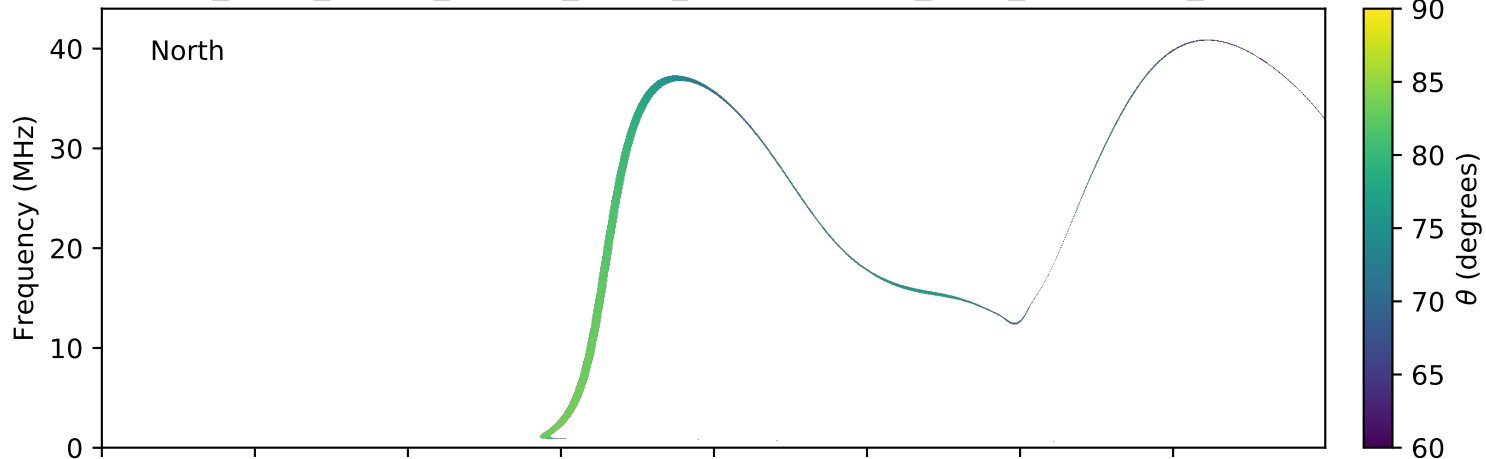
expres_earth_jupiter_europa_jrm09_lossc-wid1deg_3kev_20191209_v01.cdf
