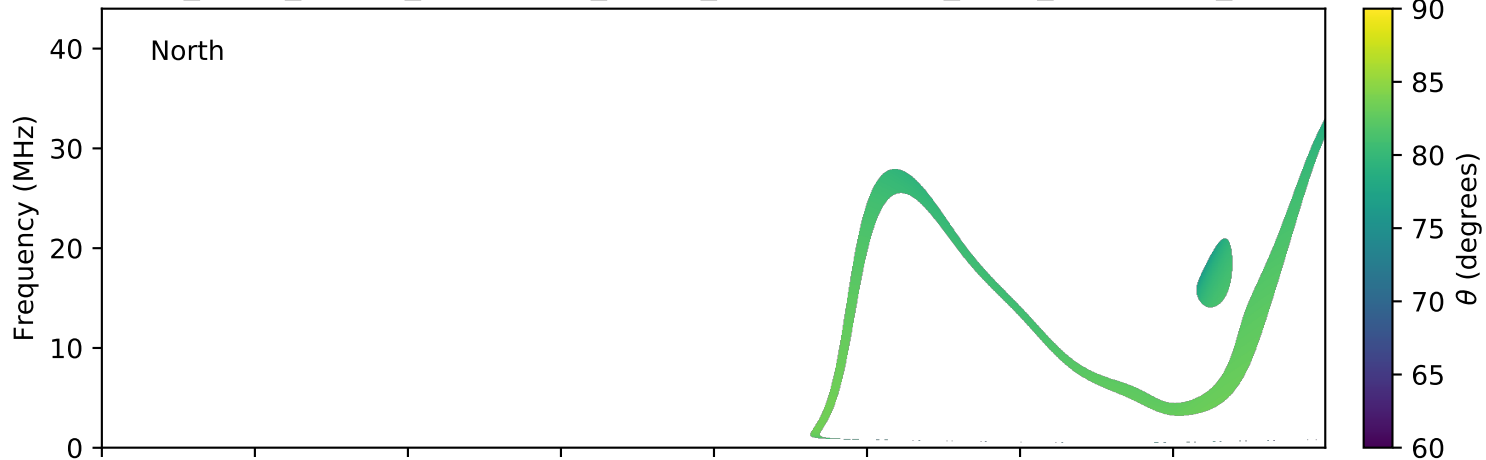
expres_earth_jupiter_ganymede_jrm09_lossc-wid1deg_3kev_20170301_v01.cdf
