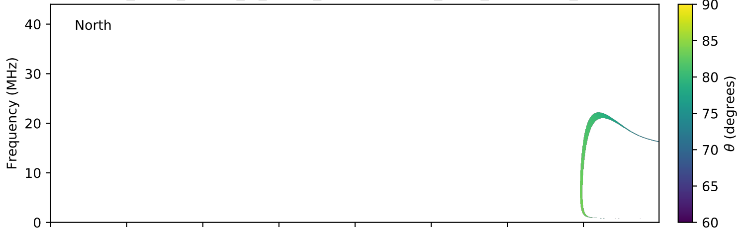
expres_earth_jupiter_io_jrm09_lossc-wid1deg_3kev_20130718_v01.cdf
