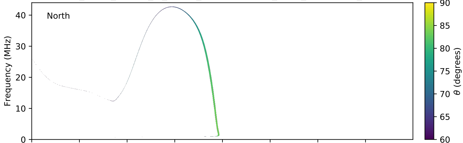
expres_earth_jupiter_io_jrm09_lossc-wid1deg_3kev_20130520_v01.cdf
