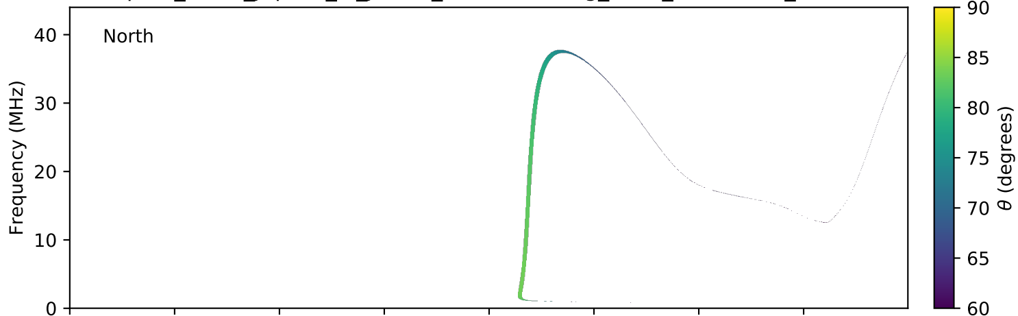
expres_earth_jupiter_io_jrm09_lossc-wid1deg_3kev_20130209_v01.cdf
