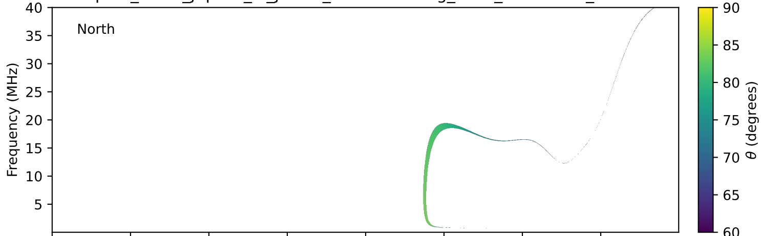
expres_earth_jupiter_io_jrm33_lossc-wid1deg_3kev_20121209_v11.cdf
