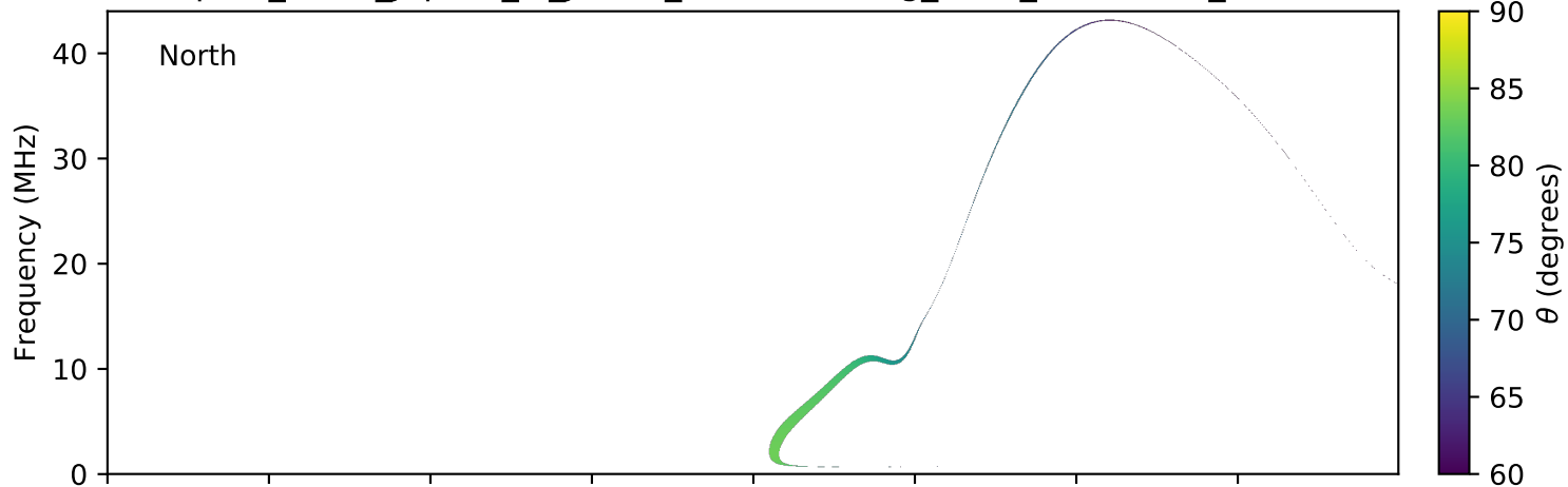
expres_earth_jupiter_io_jrm09_lossc-wid1deg_3kev_20121109_v01.cdf
