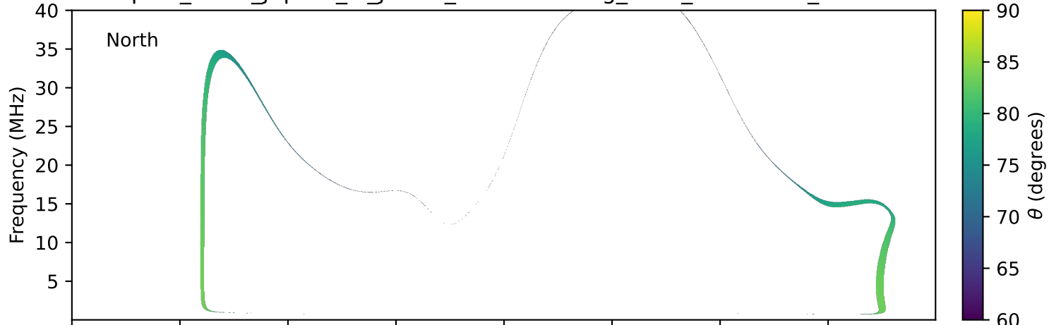
expres_earth_jupiter_io_jrm33_lossc-wid1deg_3kev_20120209_v11.cdf
