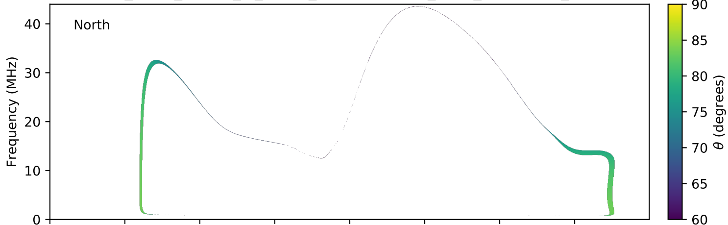
expres_earth_jupiter_io_jrm09_lossc-wid1deg_3kev_20120209_v01.cdf
