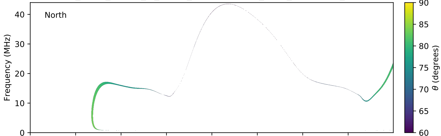
expres_earth_jupiter_io_jrm09_lossc-wid1deg_3kev_20111209_v01.cdf
