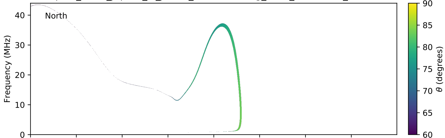
expres_earth_jupiter_io_jrm09_lossc-wid1deg_3kev_20110905_v01.cdf
