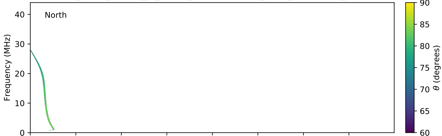
expres_earth_jupiter_io_jrm09_lossc-wid1deg_3kev_20101205_v01.cdf
