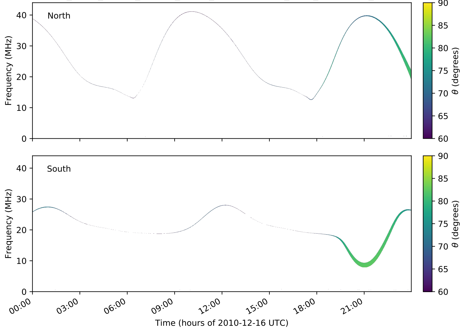
expres_earth_jupiter_europa_jrm09_lossc-wid1deg_3kev_20101216_v01.cdf
