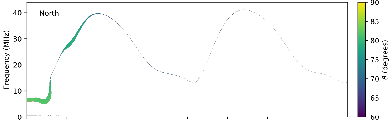
expres_earth_jupiter_europa_jrm09_lossc-wid1deg_3kev_20101212_v01.cdf
