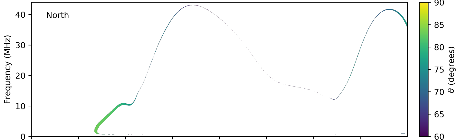
expres_earth_jupiter_io_jrm09_lossc-wid1deg_3kev_20101012_v01.cdf
