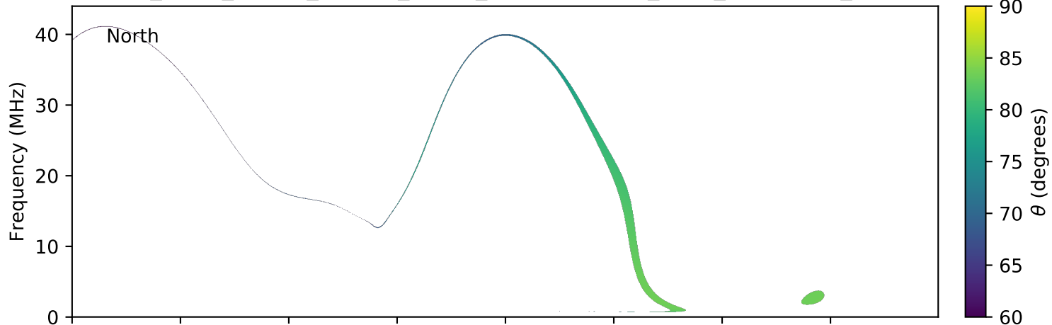
expres_earth_jupiter_europa_jrm09_lossc-wid1deg_3kev_20101017_v01.cdf
