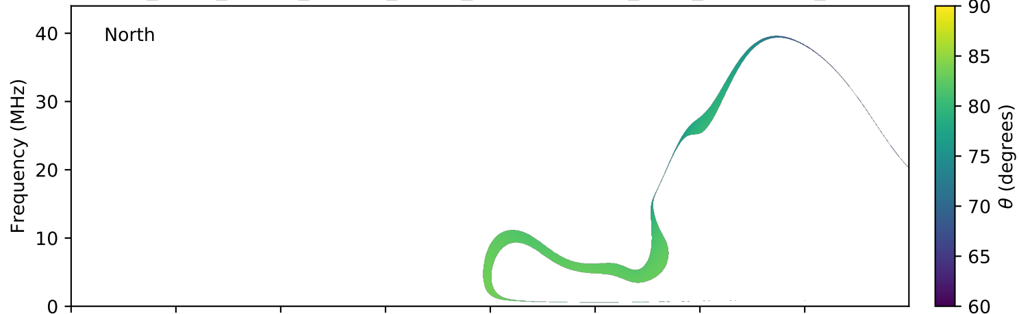
expres_earth_jupiter_europa_jrm09_lossc-wid1deg_3kev_20101012_v01.cdf
